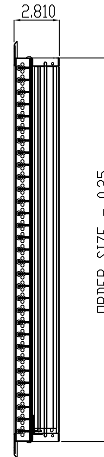
SECTION A-A SCALE 1 : 3
